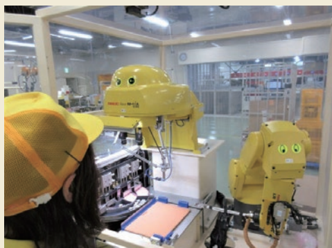
最新型「ゲンコツロボット」でキースイッチ挿入を高速で作業
