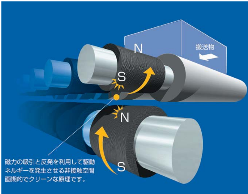
液晶テレビのガラス基板生産ラインに採用されている「レスベヤ」
